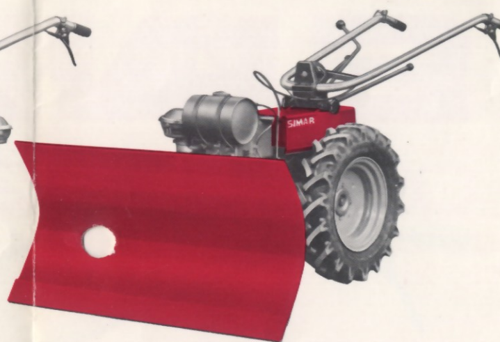
Lame à neige (Bulldozer) : largeur 0,80 m/1.10 m
