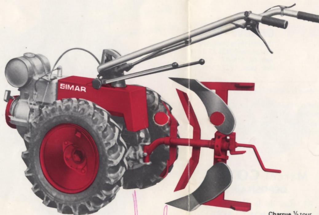
Charrue ½ tour Système de roue libre pour les virages Masses d'alourdissement
